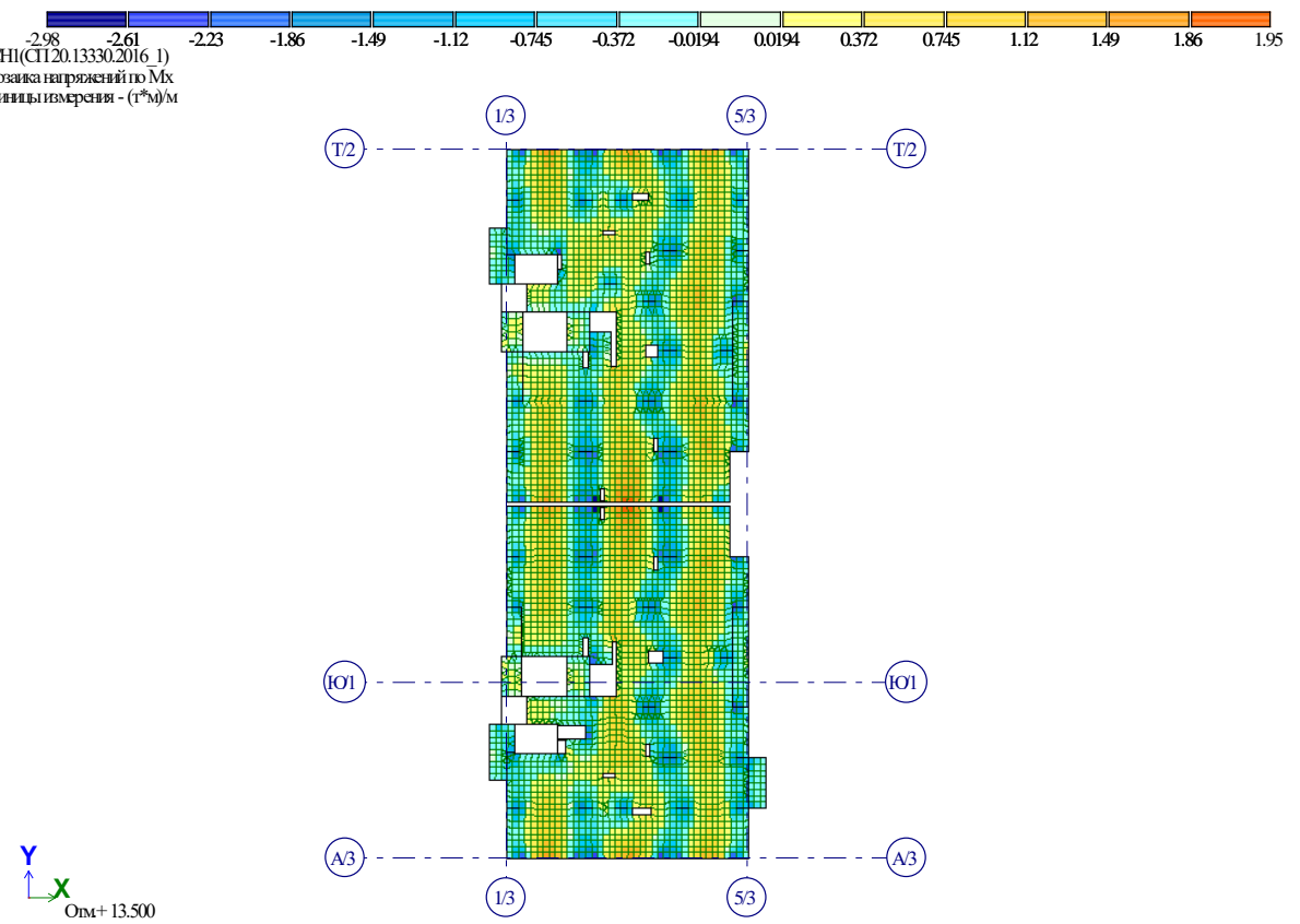
18. Рис. 9 Мозаика напряжений по Mx. Корпус 7.3
