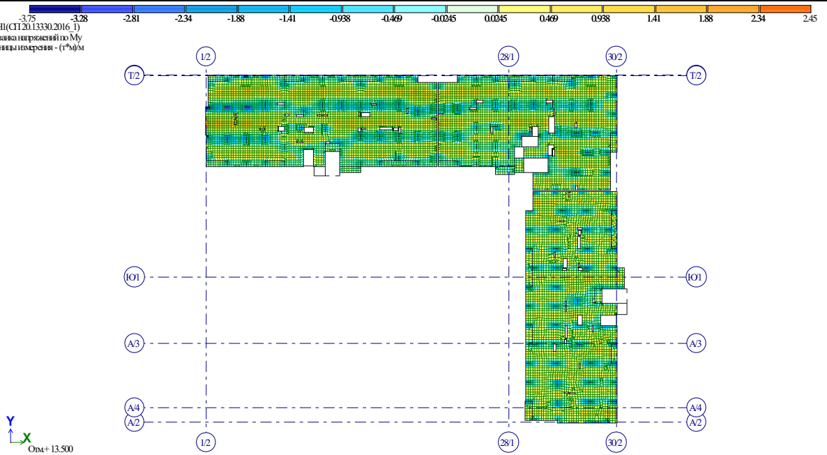
17. Рис. 8 Мозаика напряжений по My. Корпус 7.2
