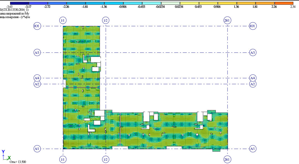
13. Рис. 6 Мозаика напряжений по Му. Корпус 7.1
