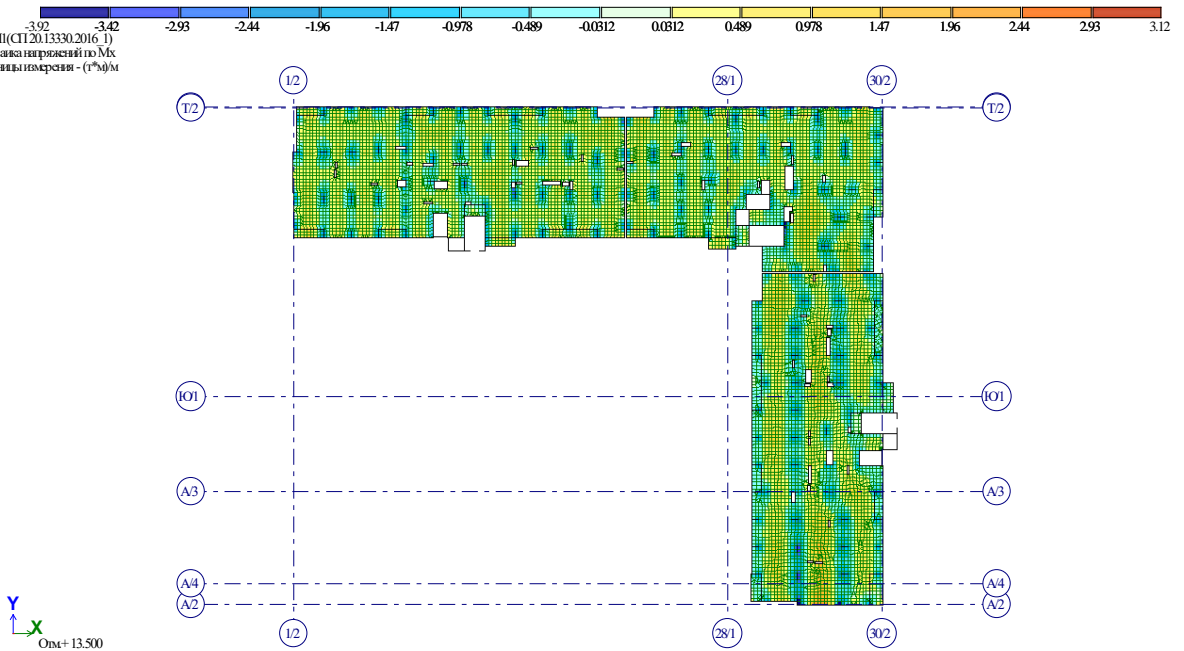
14. Рис. 7 Мозаика напряжений по Мх. Корпус 7.2
