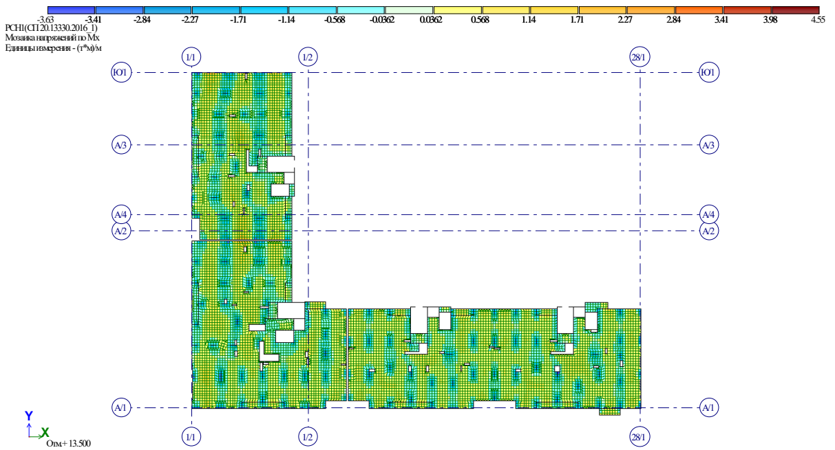
11. Рис. 5 Мозаика напряжений по Mx. Корпус 7.1
