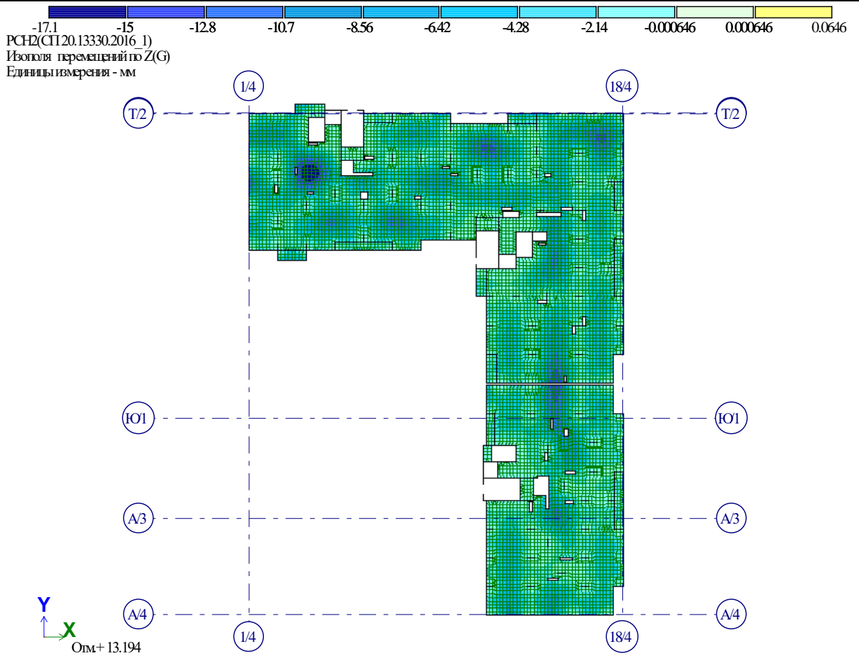
9. Рис. 4 Изополя перемещений по Z(G). Корпус 7.4
