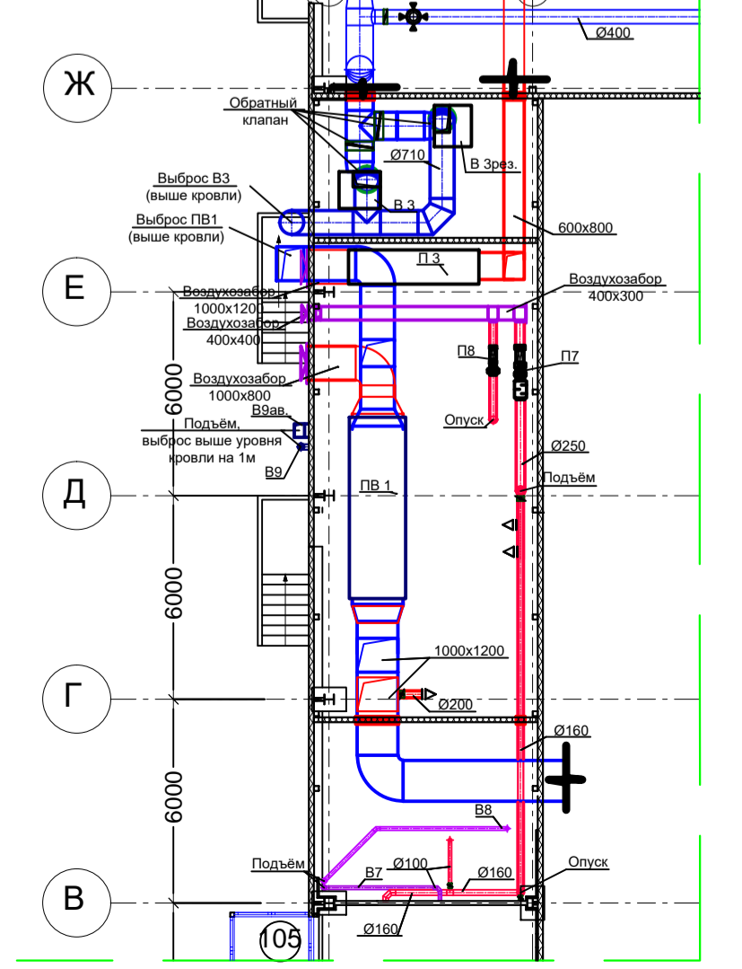
Фрагмент венткамеры на отметке +5,300
