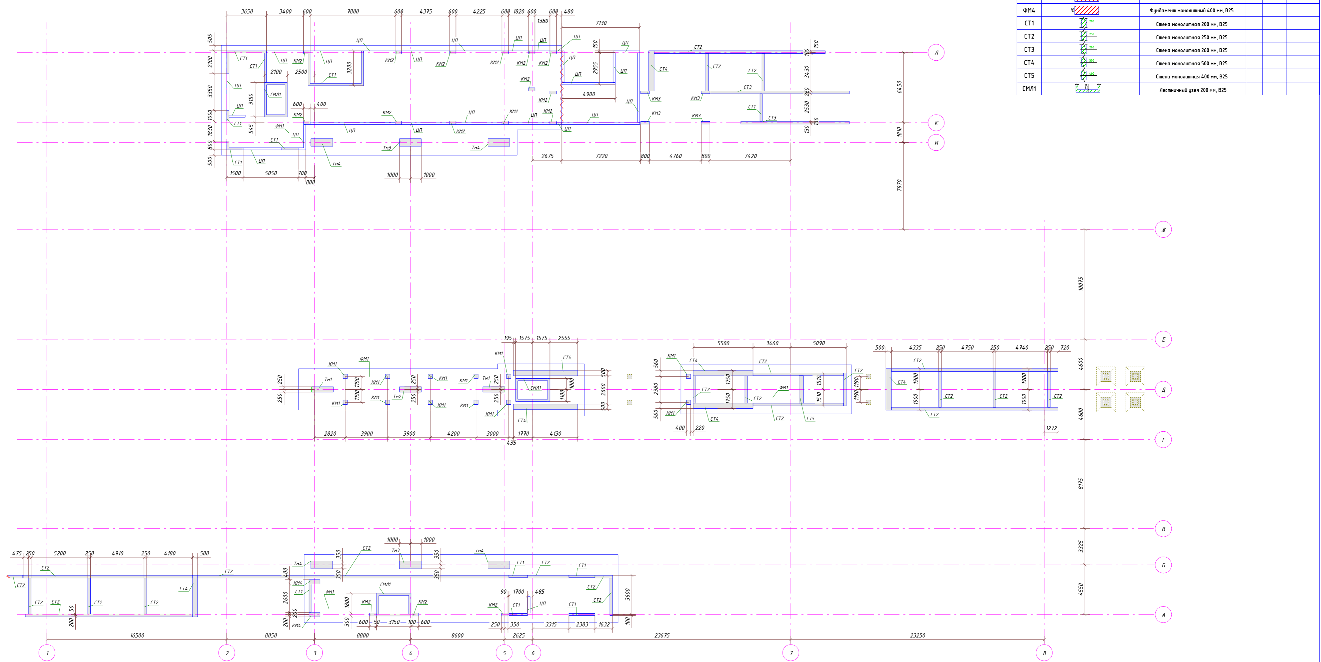
Схема расположения конструкций на отм. -10.000
