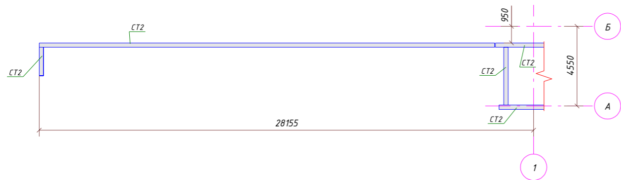
Схема расположения конструкций на отм. -10.000 подпорная стена
